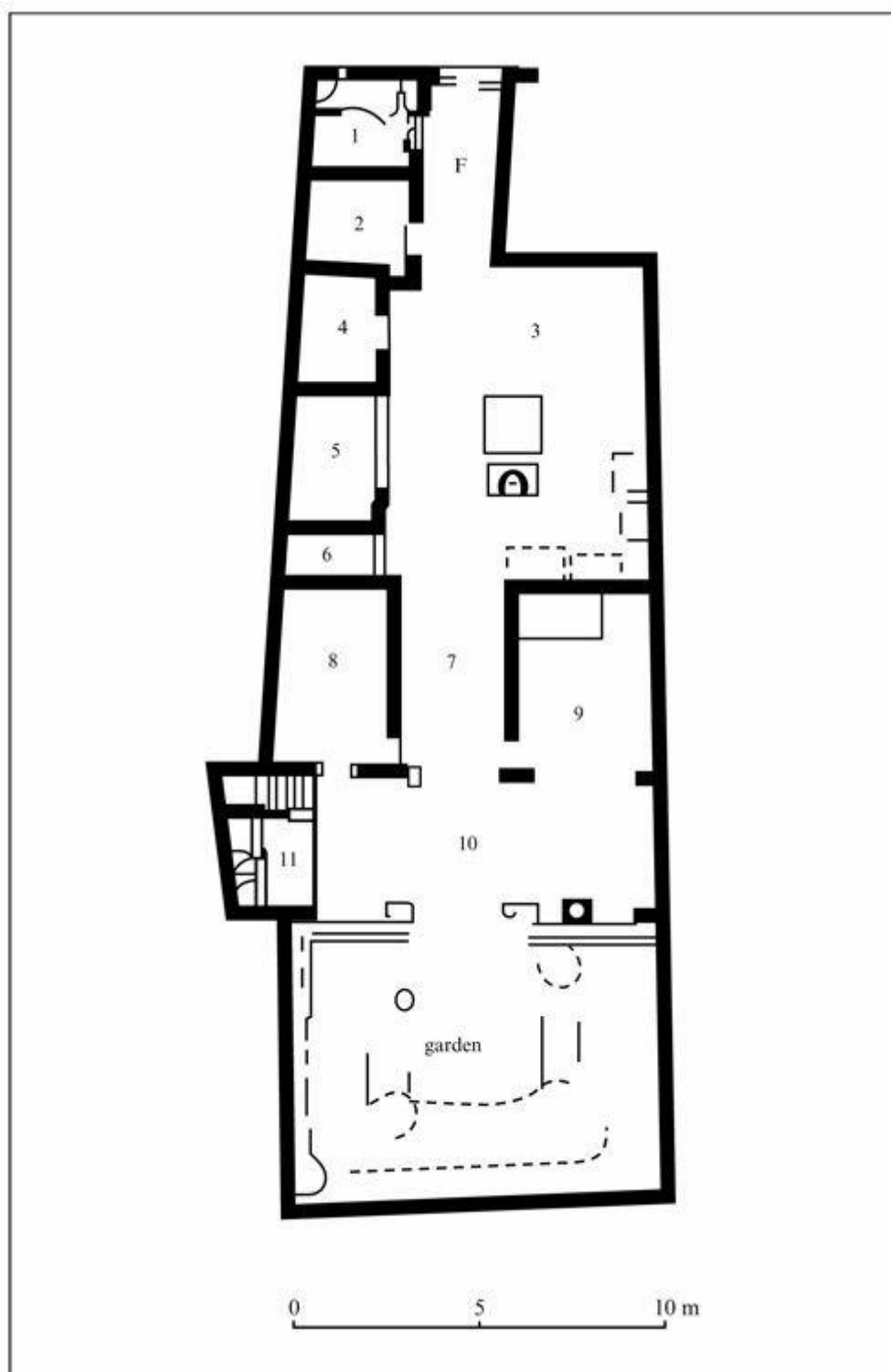
Figure 5.3. Atelier à la Casa del Fabbra à Pompéi
